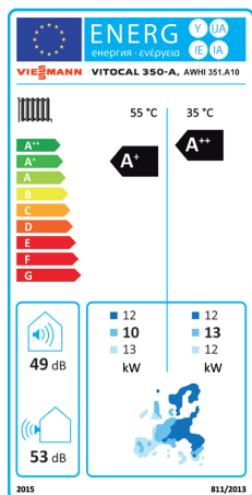
Étiquette énergétique Vitocal 350-A, AWHI 351.A10
